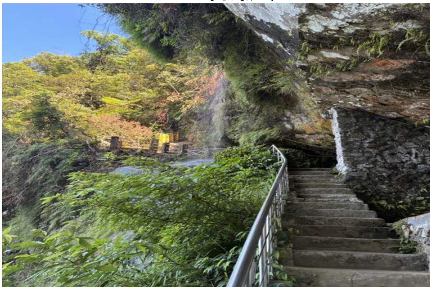
銀河洞瀑布
